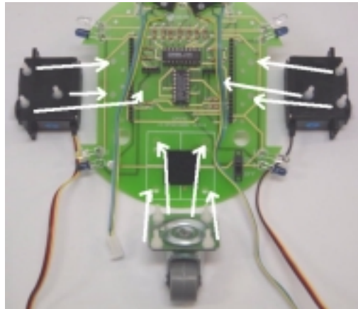
Fig. 4.19 - Motores e roda livre
