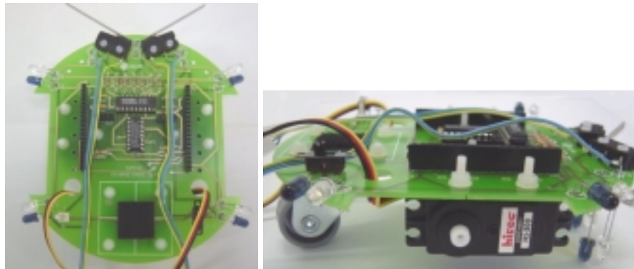
Fig. 4.20 - Montagem dos motores e roda livre
