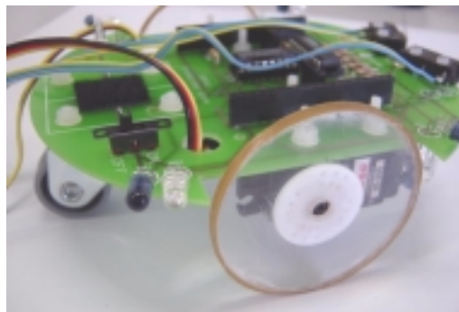
Fig. 4.21 - Montagem das rodas nos motores
